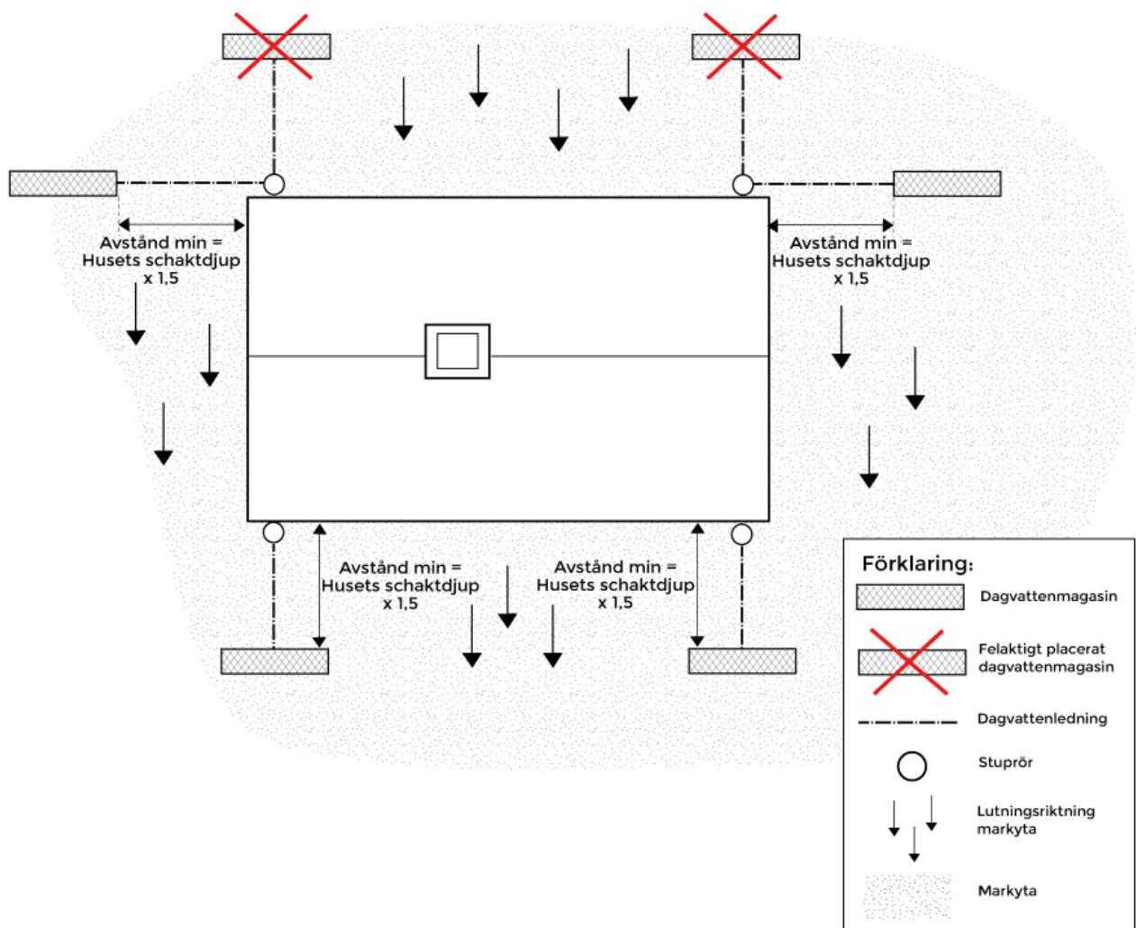
Figur 29. Placering dagvattenmagasin lutande markyta alternativ 2.
