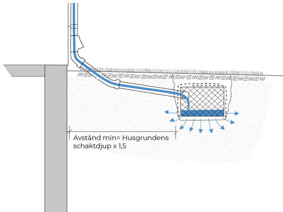
Figur 26. Placering dagvattenmagasin plan mark alternativ 1.
